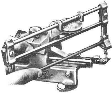
1. File-N-Joint
